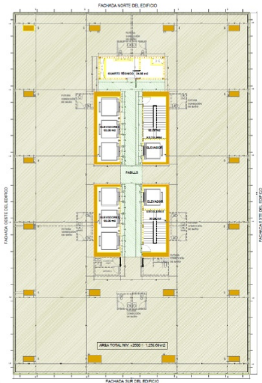
*Eti em por SIN ESCALA contrato separado y específico que refleje los términos mutuamente acordados. PLANTA ARQUITECTÓNICA - OFICINAS TORRE A - NIVEL +2500 NIVEL 34 (RIS. PÚBLICO)
